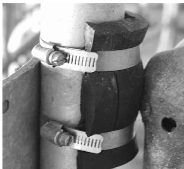
Gummimanschetten dämpfen den Lärm beim Anschlagen der Türen.
